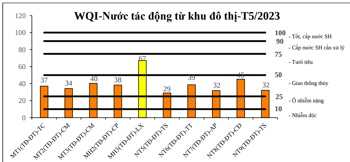
Biểu đồ 5: Diễn biến WQI khu đô thị tháng 5/2023
