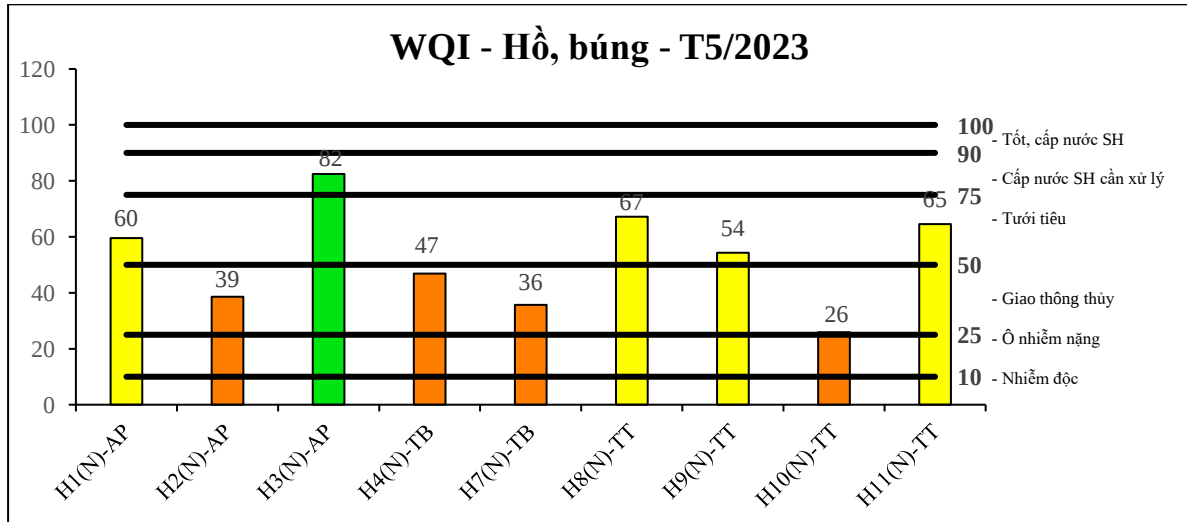
Biểu đồ 4: Diễn biến WQI hồ, búng tháng 5/2023
