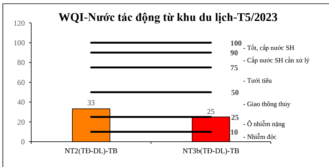
Biểu đồ 7: Diễn biến WQI khu du lịch tháng 5/2023
