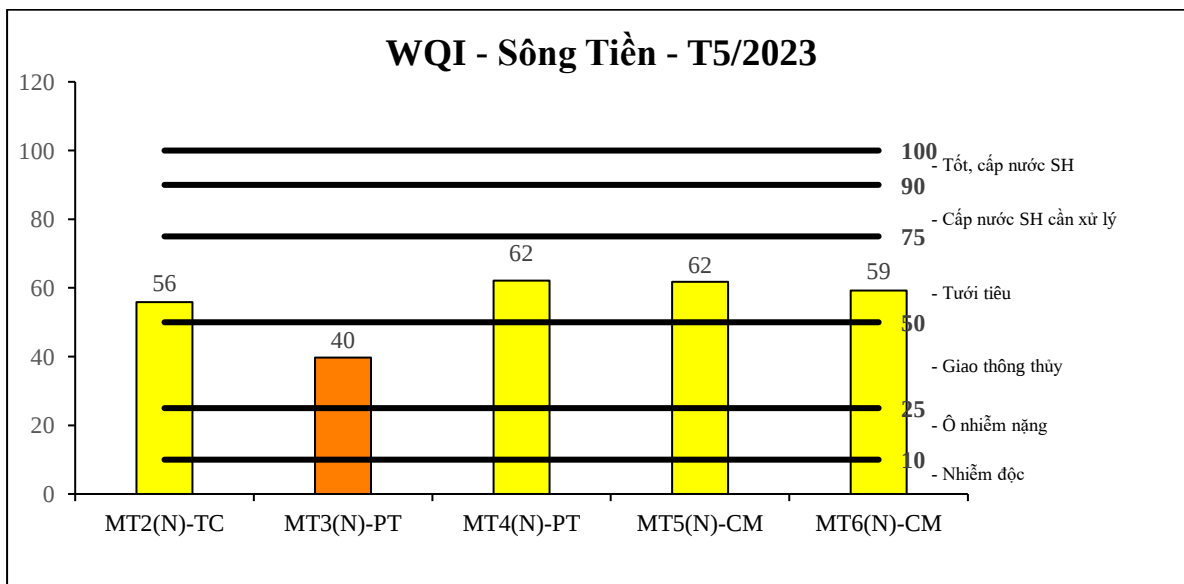
Biểu đồ 1: Diễn biến WQI đầu sông Tiền tháng 5/2023
