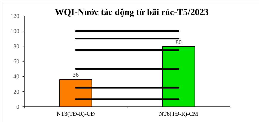
Biểu đồ 10: Diễn biến WQI nước tác động từ bãi rác đợt tháng 5/2023
