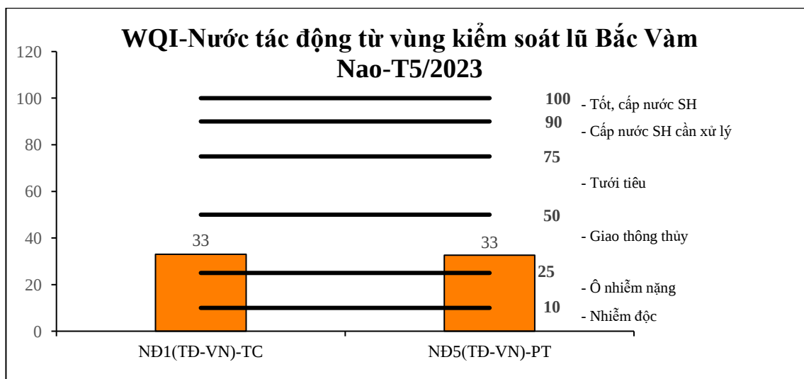
Biểu đồ 8: Diễn biến WQI khu vực Bắc Vàm Nao tháng 5/2023
