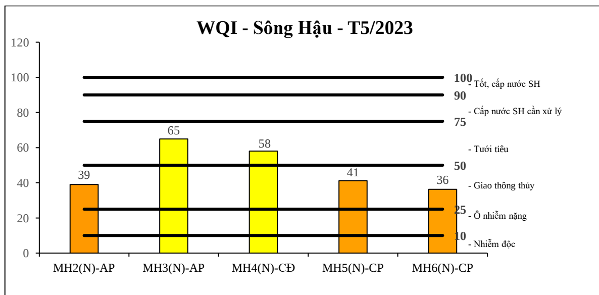
Biểu đồ 2: Diễn biến WQI s.Hậu, s.Phú Hội, s.Châu Đốc tháng 5/2023
