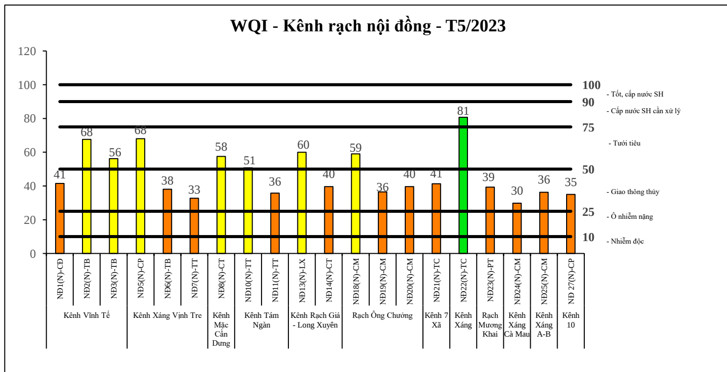
Biểu đồ 3: Diễn biến WQI kênh, rạch nội đồng tháng 5/2023
