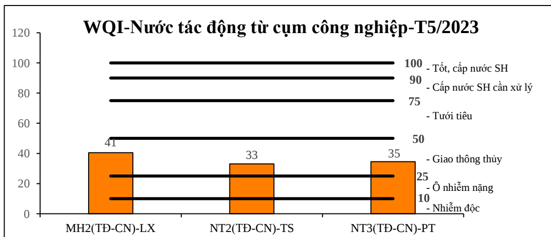
Biểu đồ 6: Diễn biến WQI cụm công nghiệp tháng 5/2023
