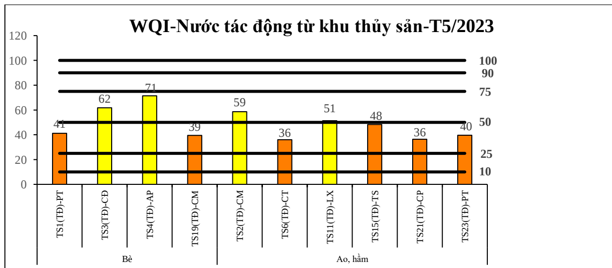
Biểu đồ 9: Diễn biến WQI khu vực nuôi trồng thủy sản tháng 5/2023
